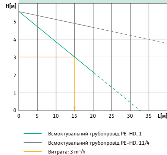
Залежність між довжиною всмоктувального трубопроводу та висотою всмоктування
