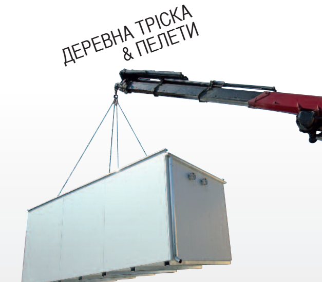
Контейнерна котельня 10 - 1 500 кВт
